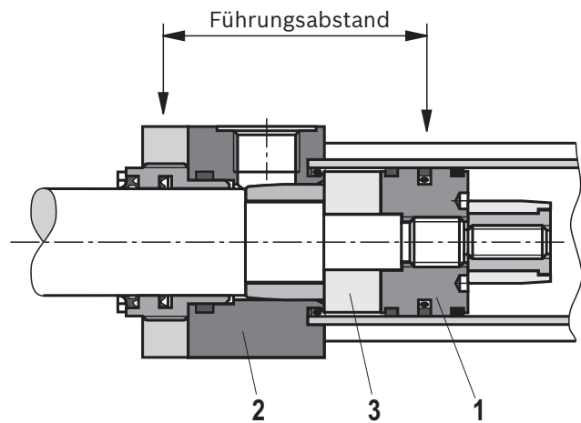
Mit Stützweitenverlängerung
