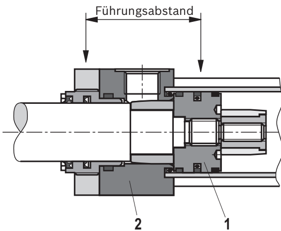
Ohne Stützweitenverlängerung
