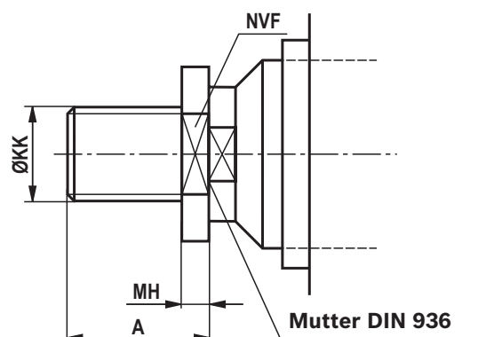
Kolbenstangenende "F"
