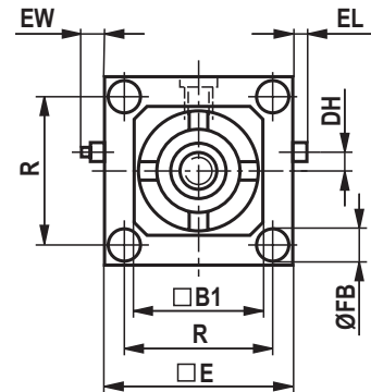
Ansicht "X" Nur für Kolben-Ø 200 mm
