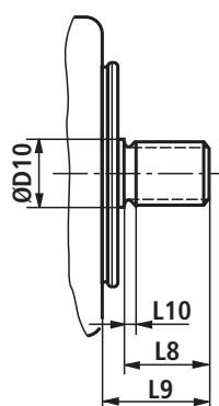
Ausführung J Vielkeilwelle SAE-B oder C
