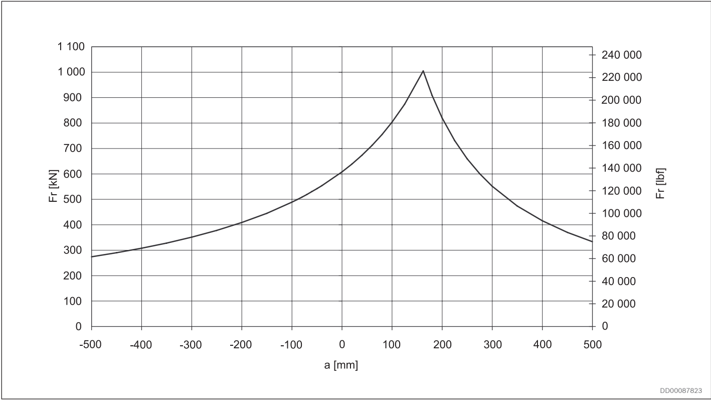
Fig. 64: Permissible external static load Hägglunds CB 400
