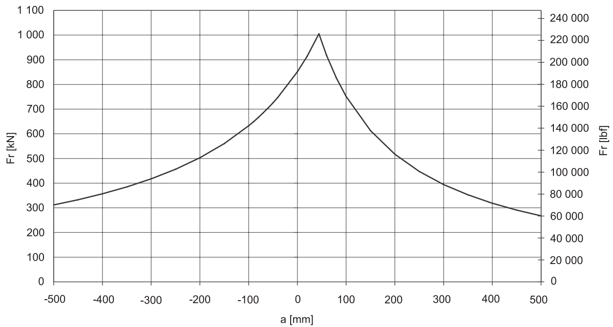
Fig. 65: Permissible external static load Hägglunds CB 560
