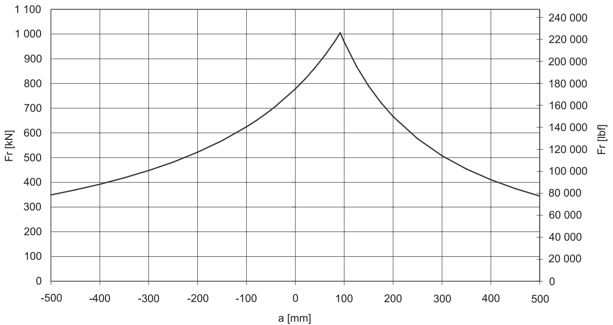
Fig. 66: Permissible external static load Hägglunds CB 840
