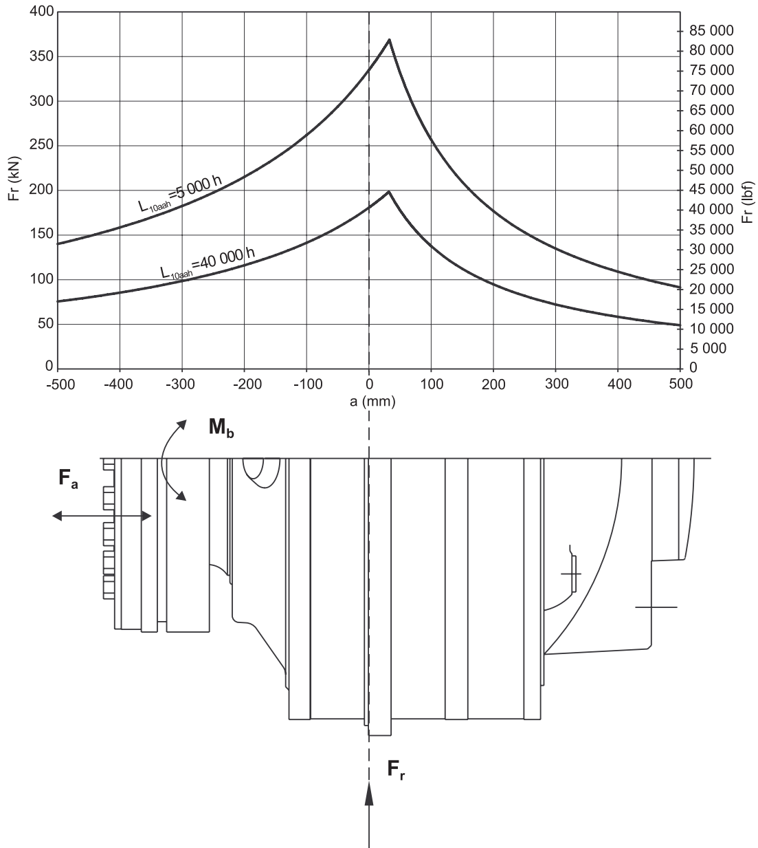
Fig. 61: Permissible external dynamic loads Hägglunds CB 840
