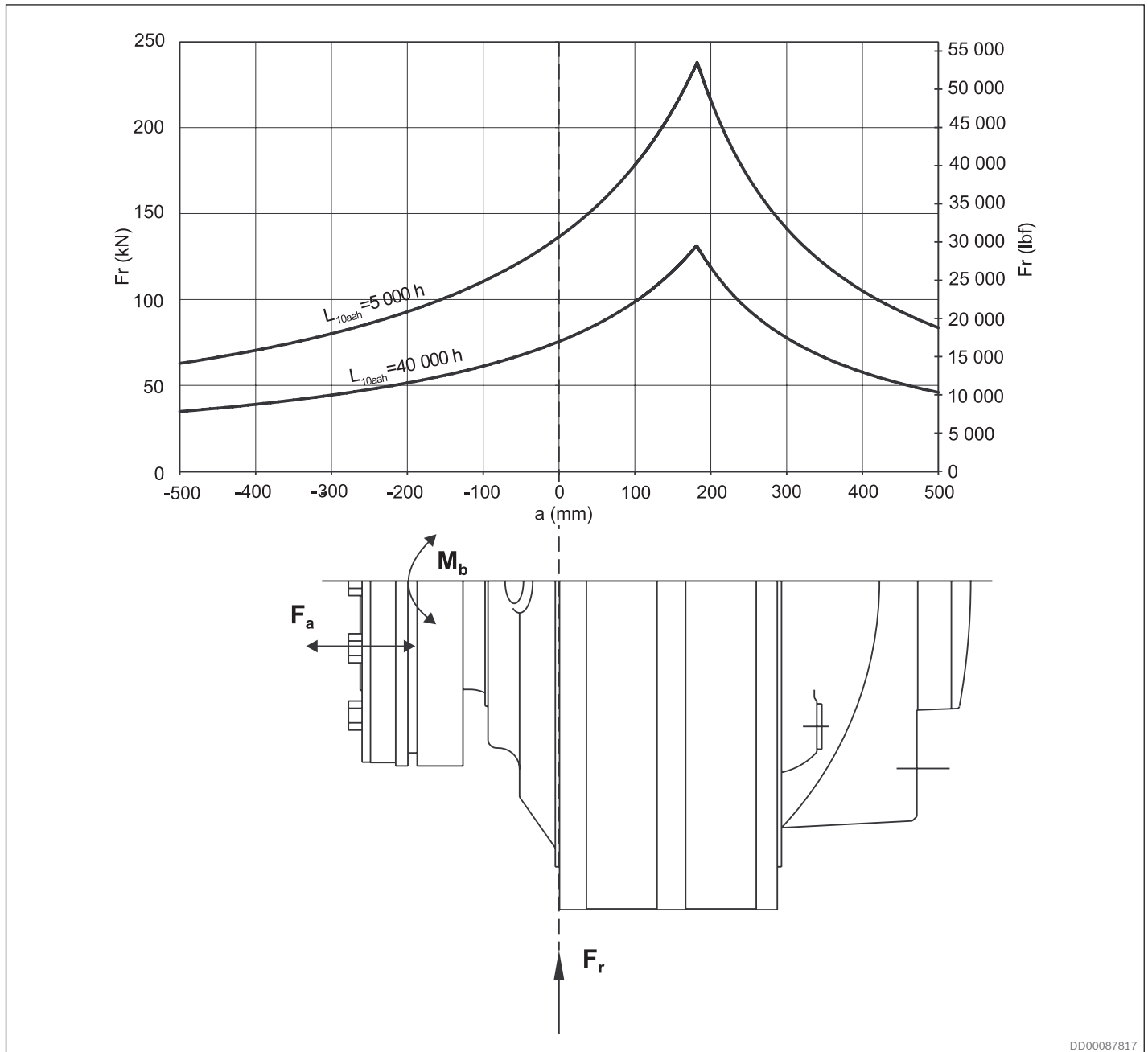
Fig. 59: Permissible external dynamic loads Häggblunds CB 400
