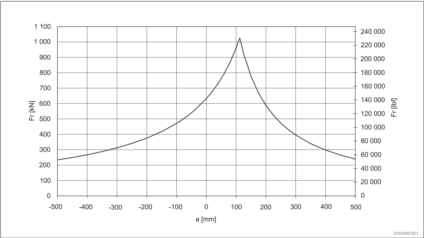
Fig. 63: Permissible external static load Hägglunds CB 280
