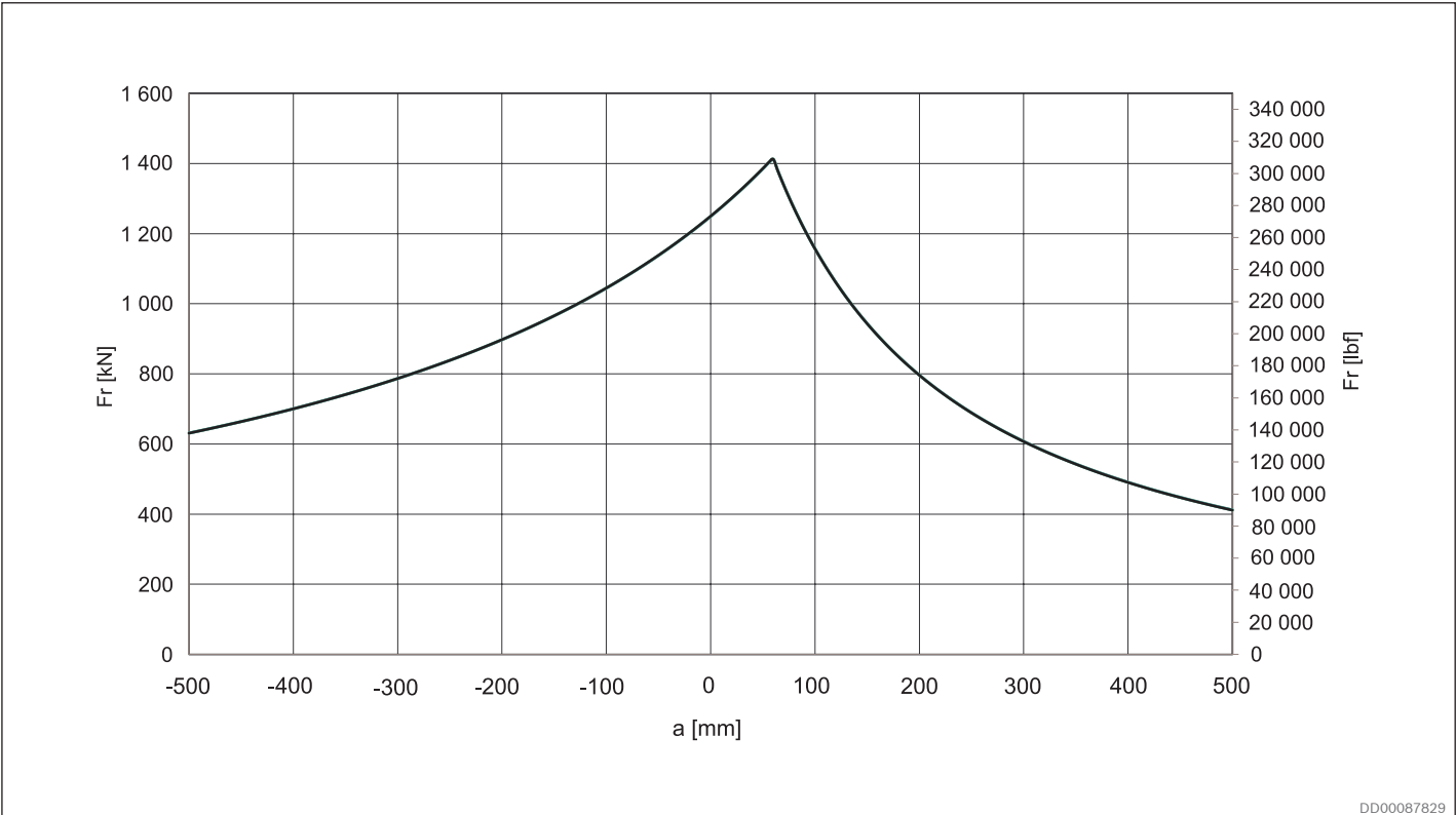
Fig. 67: Permissible external static load Hägglunds CB 1120
